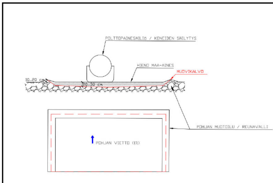
Kuva y. Maaperäsuojauksen periaatepiirros
