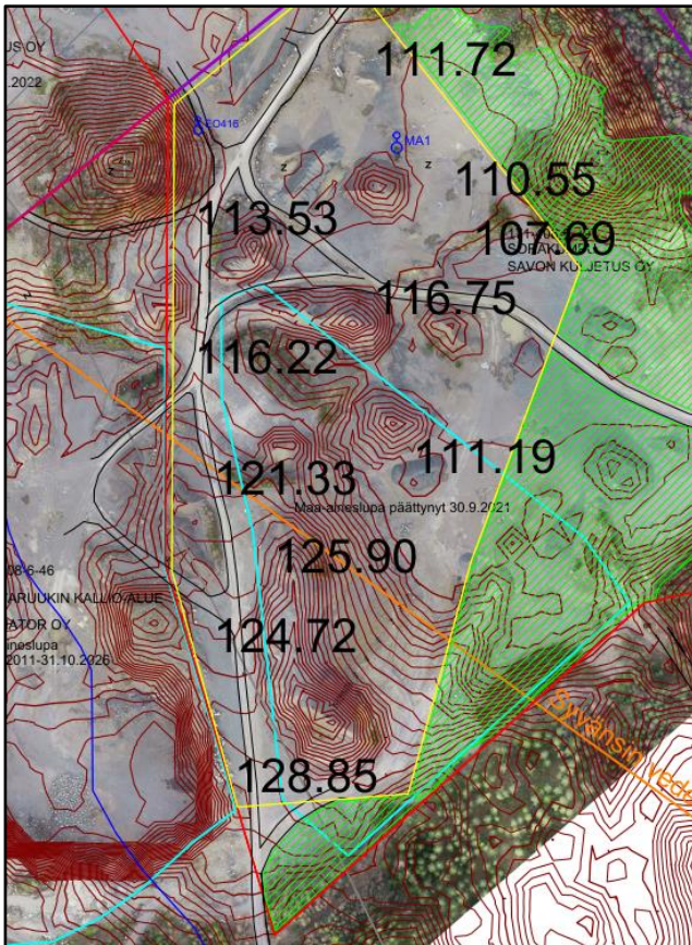
Kuva 1. Varastointialueella olevien korkeuspisteiden arvoja (N2000) syksyllä 2020 mitatun korkeusaineiston mukaan.
