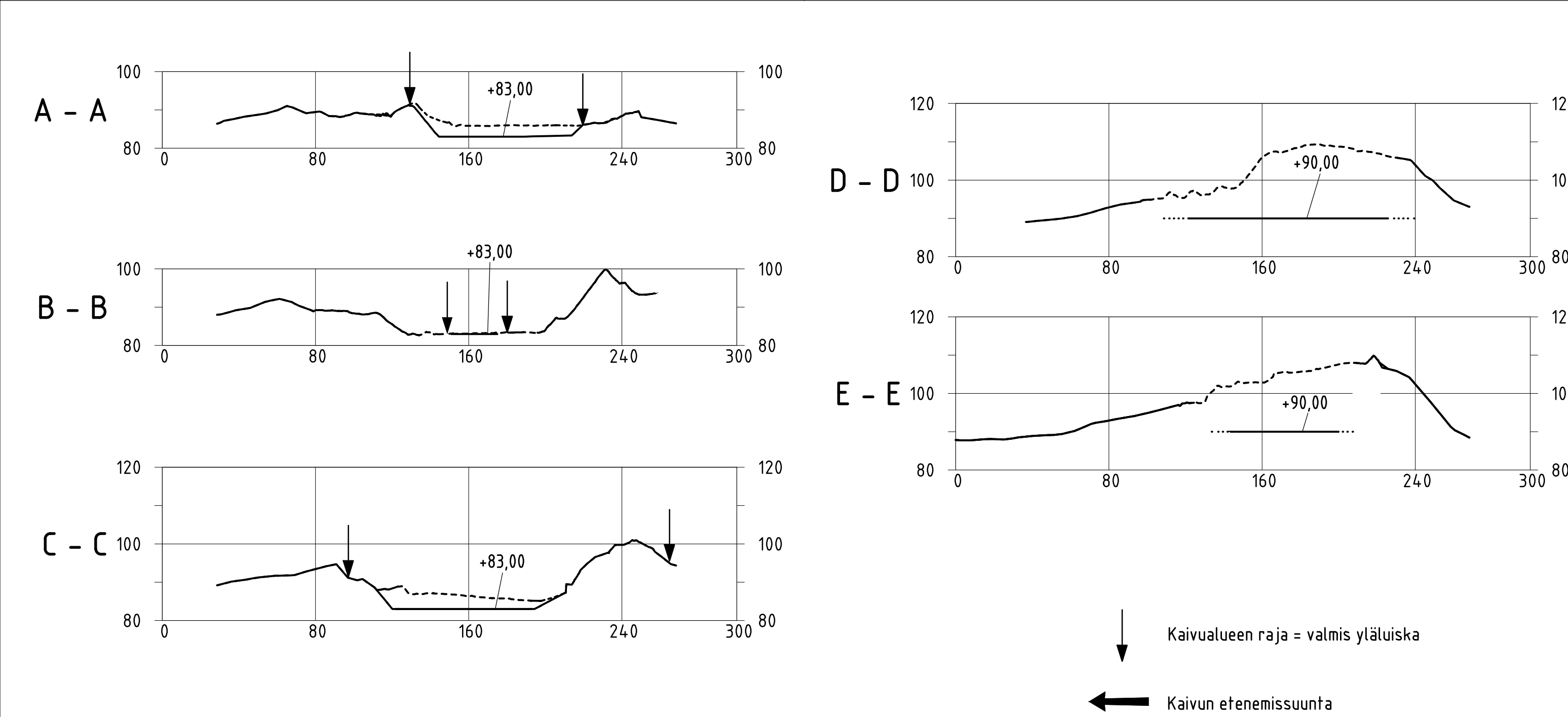
Leikkaukset 1:2000 / 1:1000 Kaikki ulkoreunojen luiskat muotoillaan kaltevuuteen 1:2
